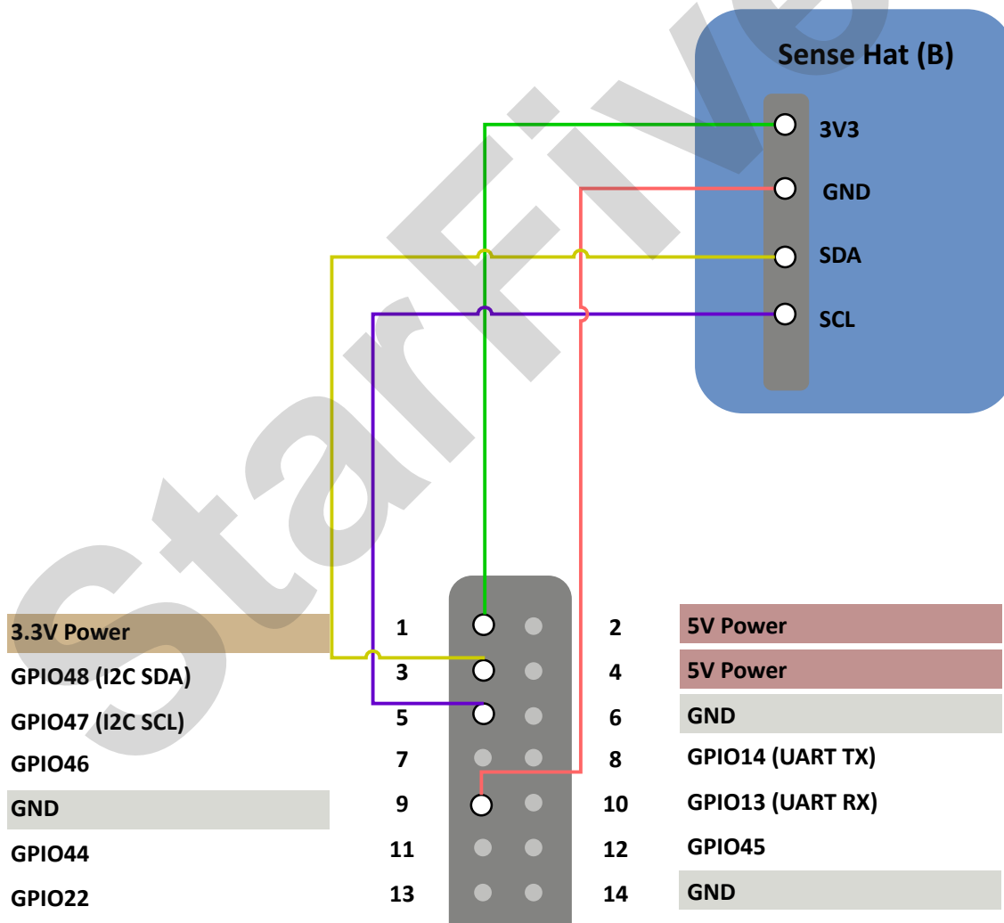
图 2-1 将Sense Hat (B)连接到40-Pin Header上
